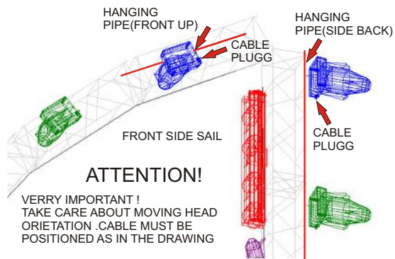
RAČUNALNI NACRT DETALJA ZA MONTAŽU RASVJETE
